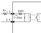
CW(Pin:1,2), CCW(Pin:3,4)
